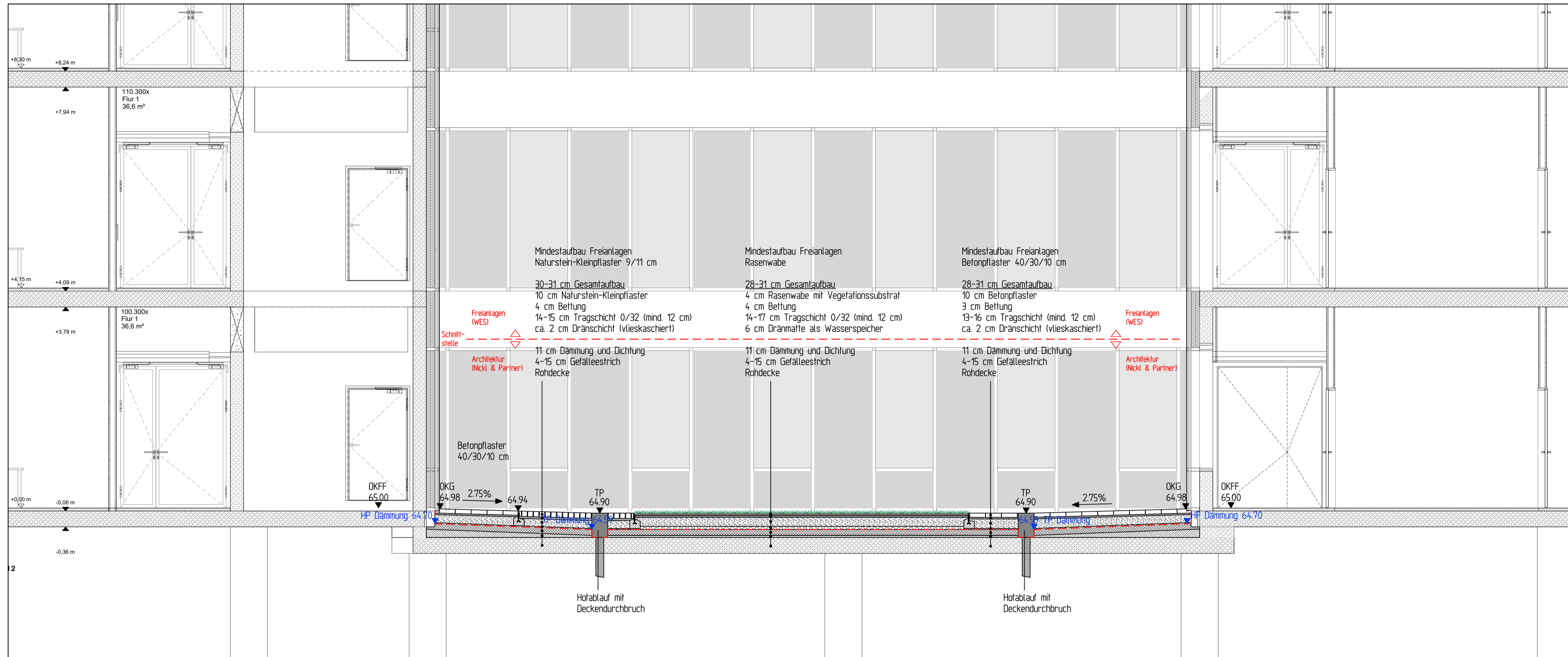
Schnitt Innenhof AA; MedForCe Bauteil C M150
