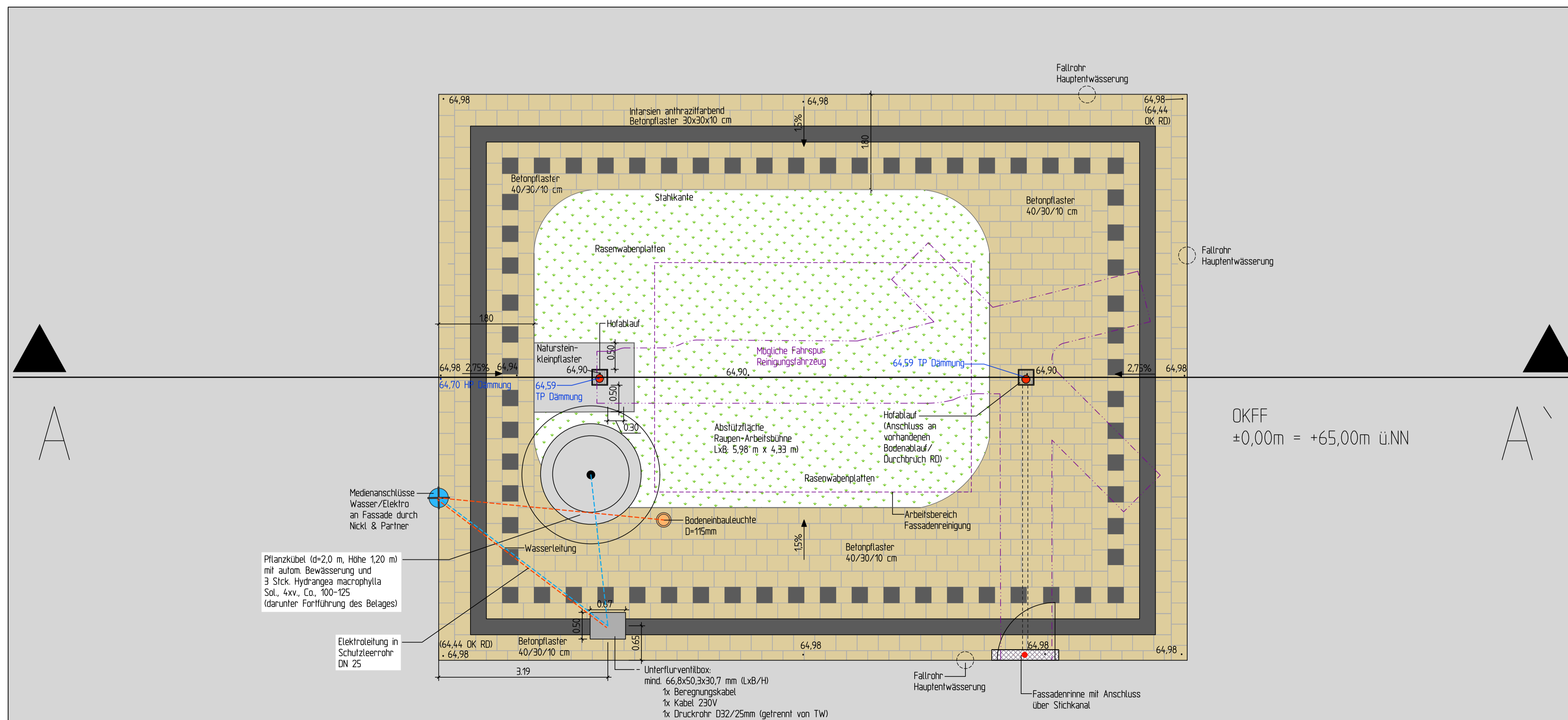
Detailausschnitt Innenhof; MedForCe Bauteil C M150
